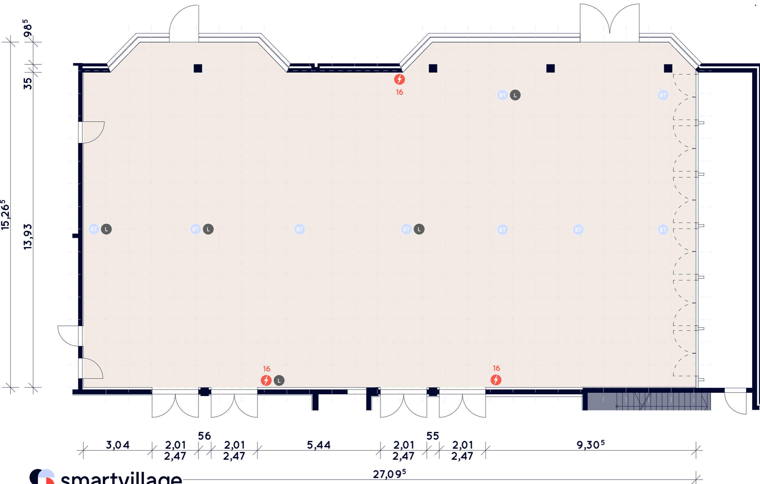
LAGEPLAN
